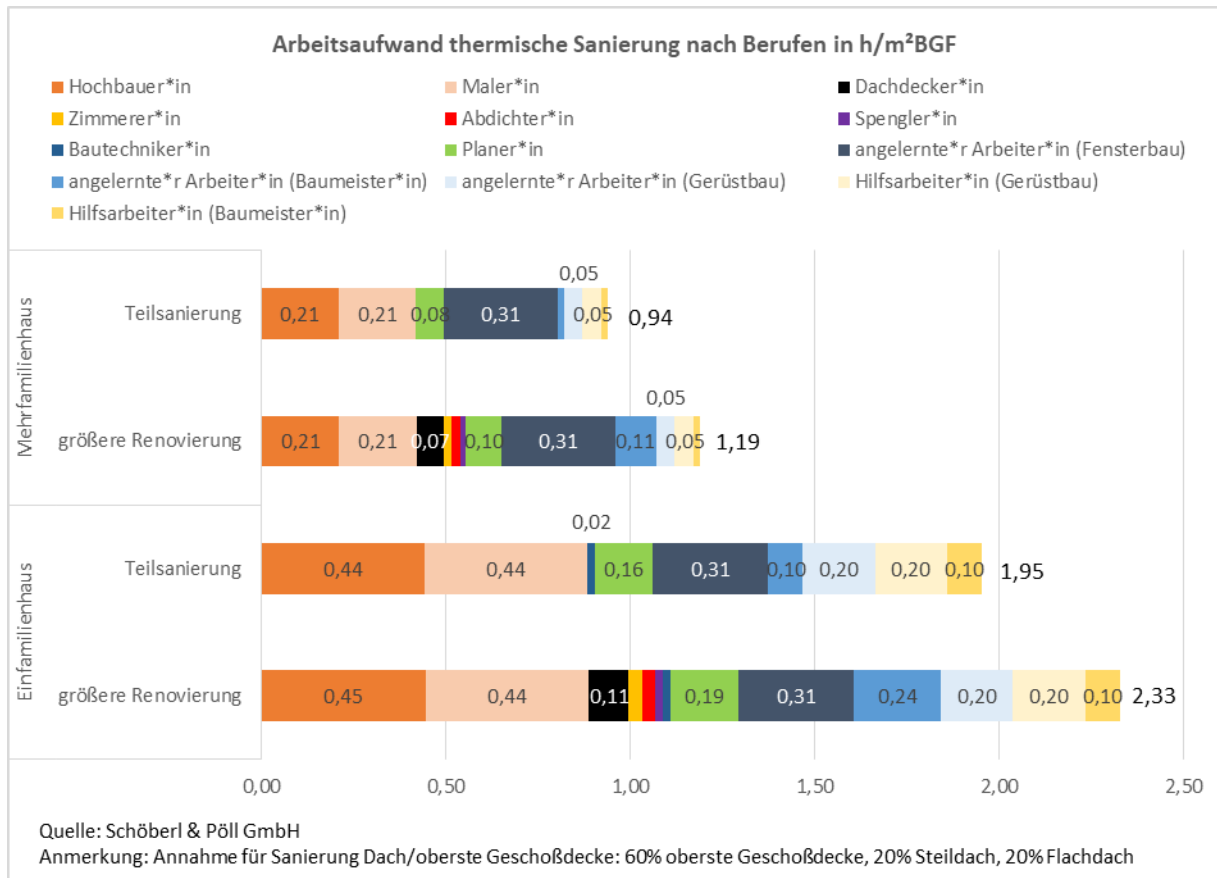
Abbildung 17 Arbeitsaufwand thermische Sanierung nach Berufen in h/m 2 BGF
